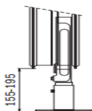
Console indépendante Montage au sol
